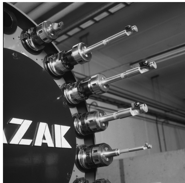
Errix-Werkzeuge in einem NC-Magazin
